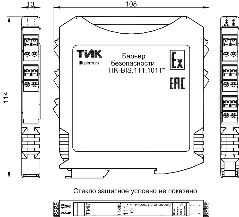
Рисунок 5 – Внешний вид и габаритные размеры барьеров безопасности ТИК-BIS.111.1X1X
