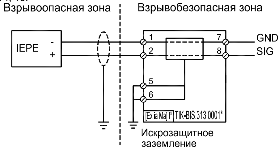
Рисунок 14 – Схема подключения барьеров безопасности ТИК-BIS.313.0X0X
