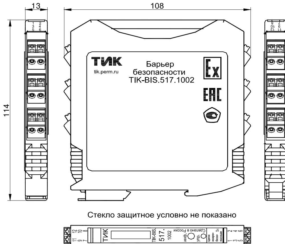
Рисунок 18 – Внешний вид и габаритные размеры барьера безопасности ТИК-BIS.517.1002
