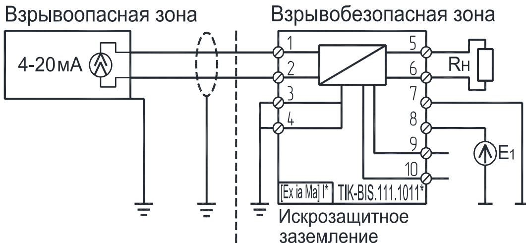
Рисунок 6 – Схема подключения барьеров безопасности ТИК-BIS.111.1X1X активный выход
