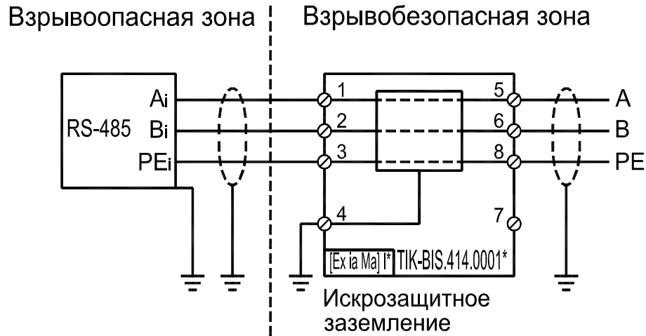
Рисунок 17 – Схема подключения барьеров безопасности ТИК-BIS.414.000X
