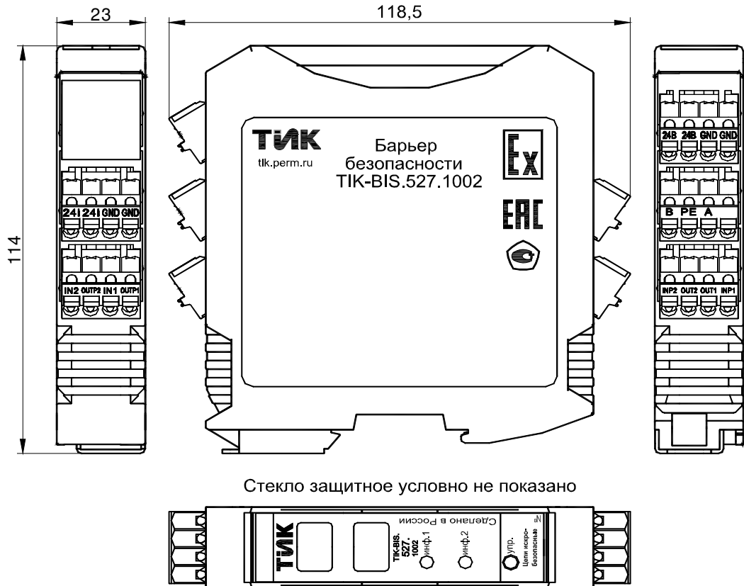
Рисунок 20 – Внешний вид и габаритные размеры барьера безопасности ТИК-BIS.527.1002
