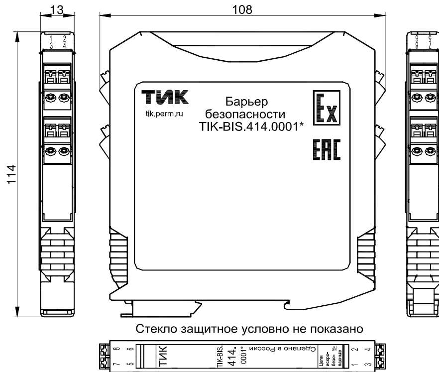
Рисунок 16 – Внешний вид и габаритные размеры барьеров безопасности ТИК-BIS.414.000X
