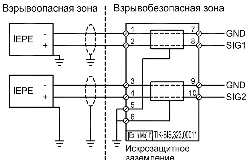
Рисунок 15 – Схема подключения барьеров безопасности ТИК-BIS.323.0X0X
