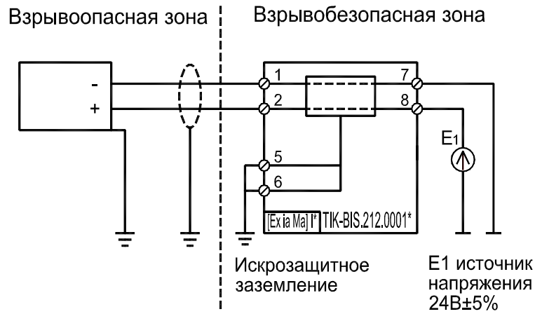
Рисунок 10 –Схема подключения барьеров безопасности ТИК-BIS.212.0X0X
