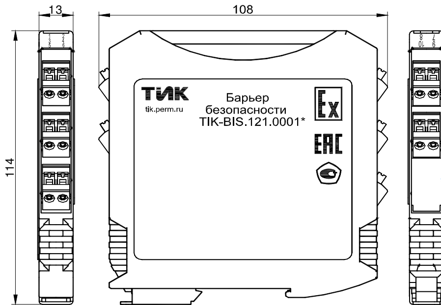
Рисунок 1 – Внешний вид и габаритные размеры барьеров безопасности ТИК-BIS.111.0X0X
