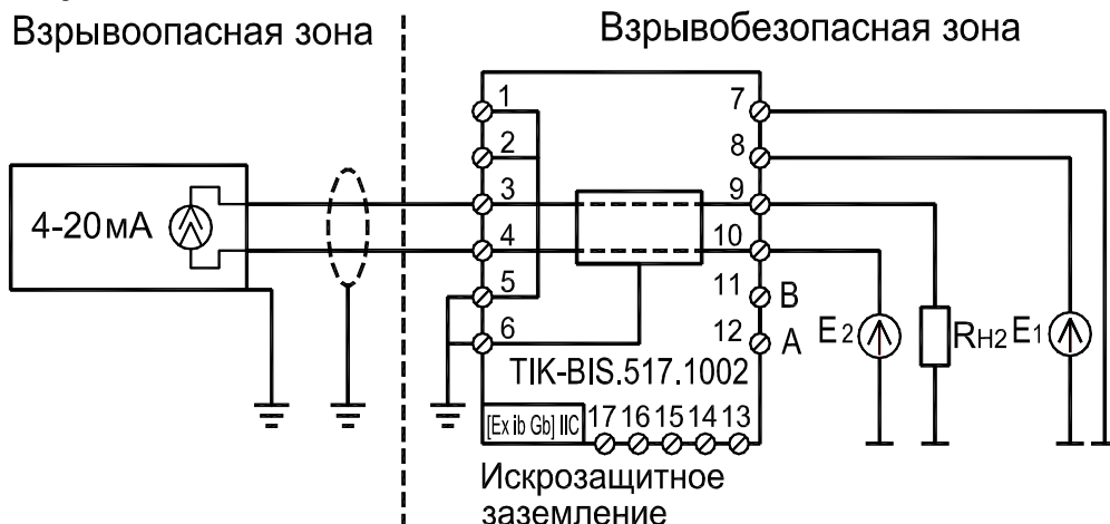
Рисунок 19 – Схема подключения барьера безопасности ТИК-BIS.517.1002
