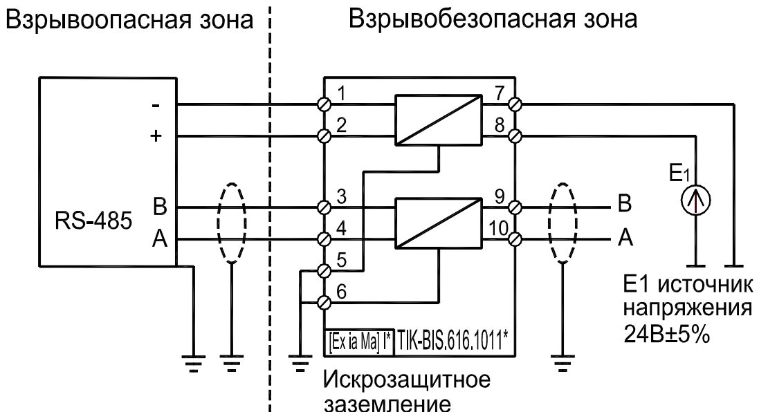
Рисунок 24 – Схема подключения барьеров безопасности ТИК-BIS.616.1X1X
